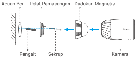
Gambar 1 Pemasangan dengan Dudukan Magnetis
